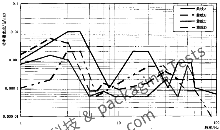
图 A.2 不同荷载卡车随机振动 PSD 曲线
