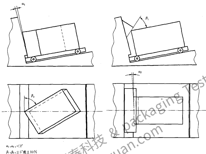
a) 对一垂直棱的冲击 b) 对一水平棱的冲击
